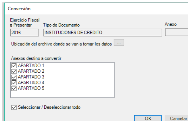
Ventana de Conversión de DISIF. (Fig. 239.)
